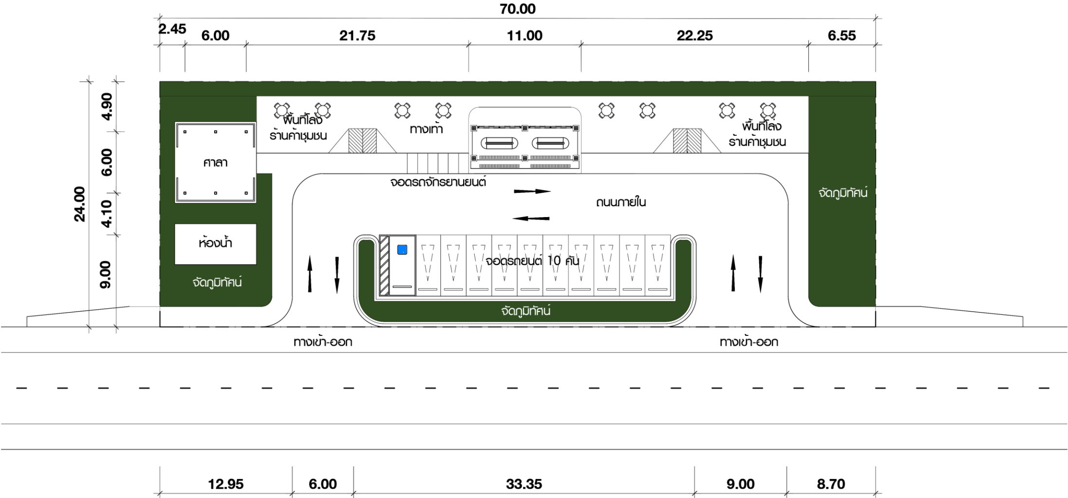
ผังบริเวณจุดชมวิวขนาดกลาง
